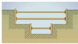
Figura 7 - Escavação tabuleada (escavação com paredes em tabuleado).
