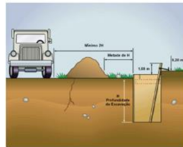
Figura 3 - Medidas de afastamento mínimo convenientemente adotadas.
